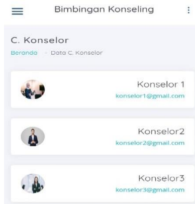
Gambar 5. Halaman Konselor
